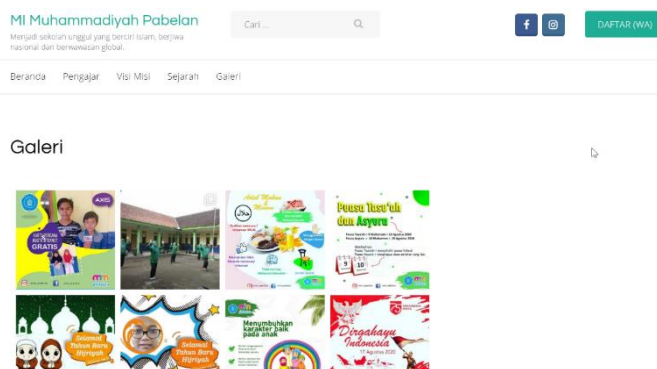
Gambar 8 Tampilan Galeri
