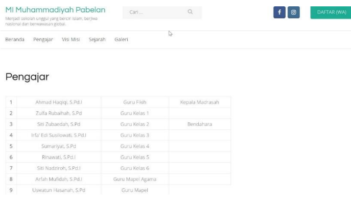
Gambar 7 Tampilan Pengajar
