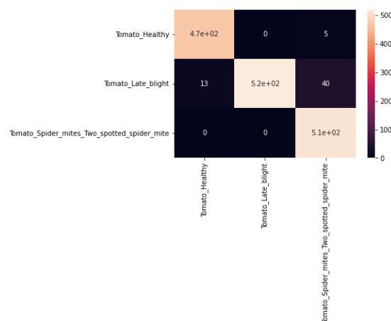
Figure 9. Confusion Matrix SA
